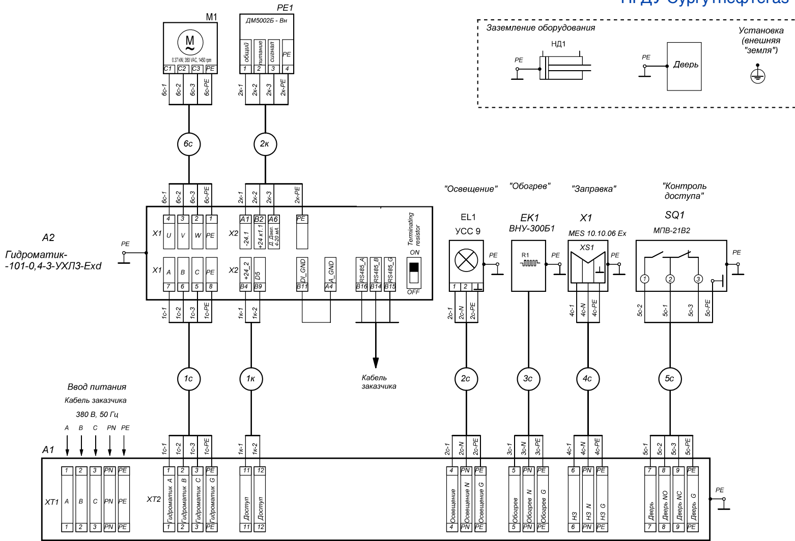
Рис.4д. Схема внешних подключений. (С цифровым манометром DM5002)
