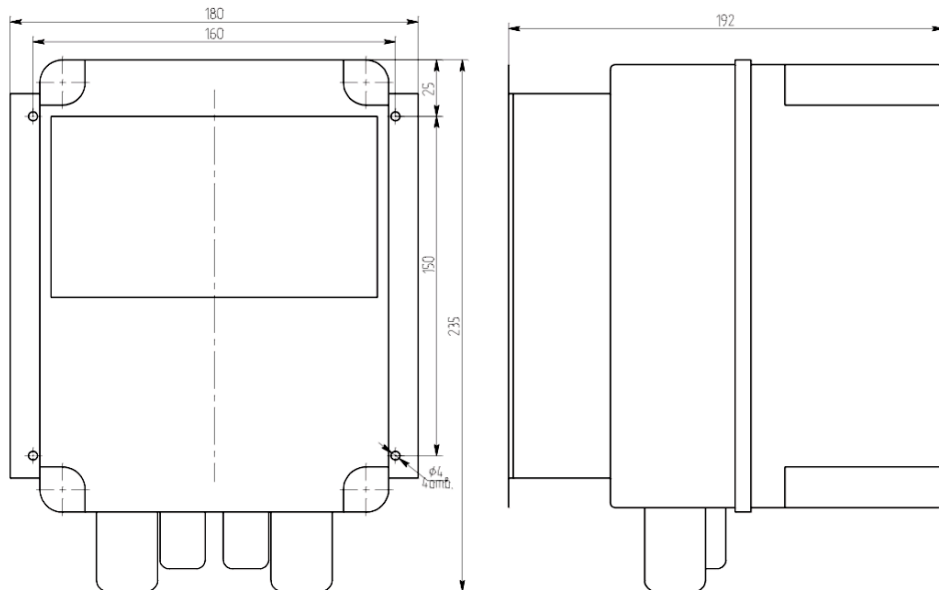
Габаритные и установочные размеры БУДН-05-5,5 ÷ 11
