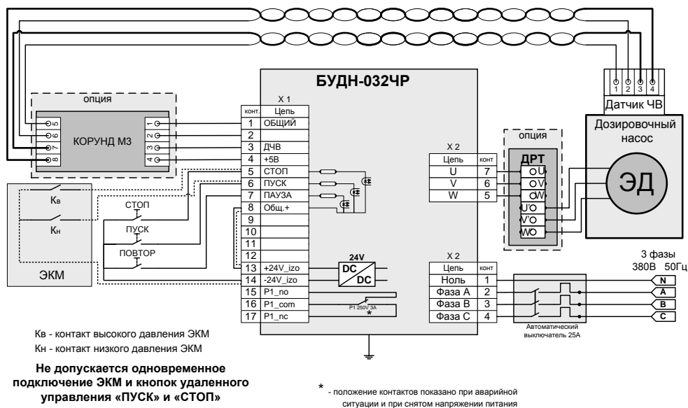
Рисунок 11 – Вариант монтажной схемы подключения БУ с использованием внешних кнопок «ПУСК», «СТОП», «ПОВТОР» и ЭКМ и встроенного источника питания.
