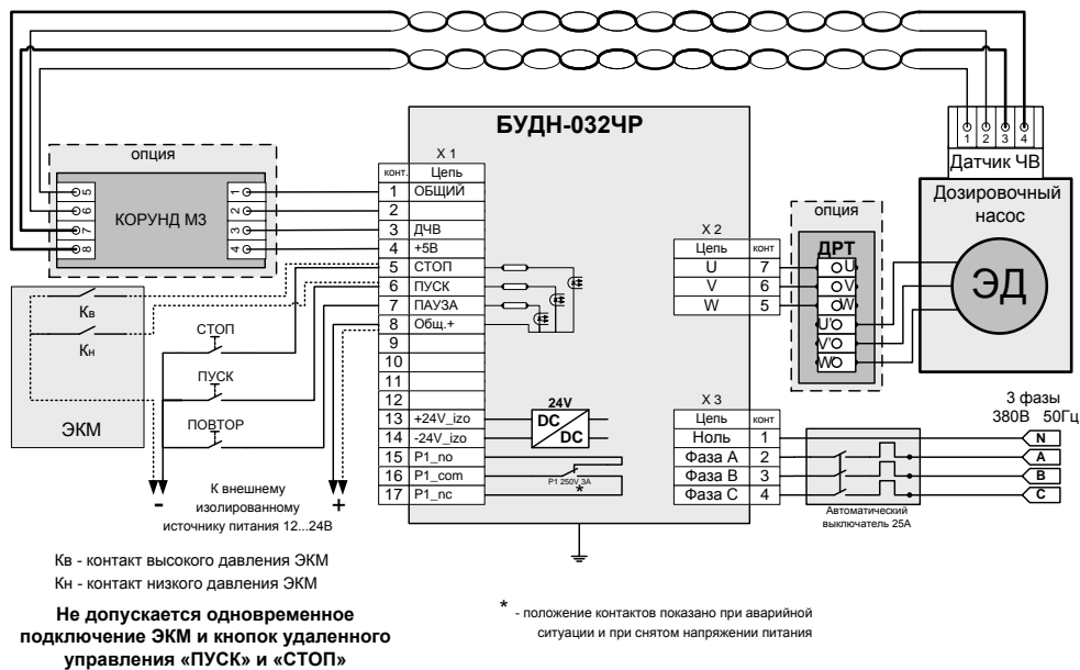
Рисунок 10 – Вариант монтажной схемы подключения БУ с использованием внешних кнопок «ПУСК», «СТОП», «ПОВТОР» и ЭКМ.
